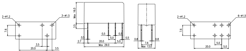
RQ2/RQ1 HC
