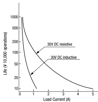
(RY4)
