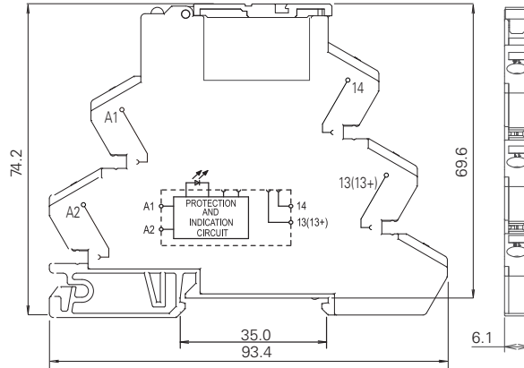
RV8S-S Spring Clamp Terminal (mm)
