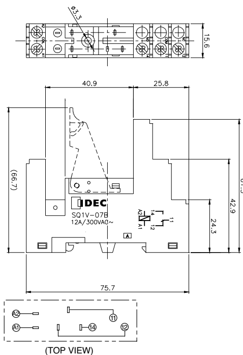
SQ1V-07B
