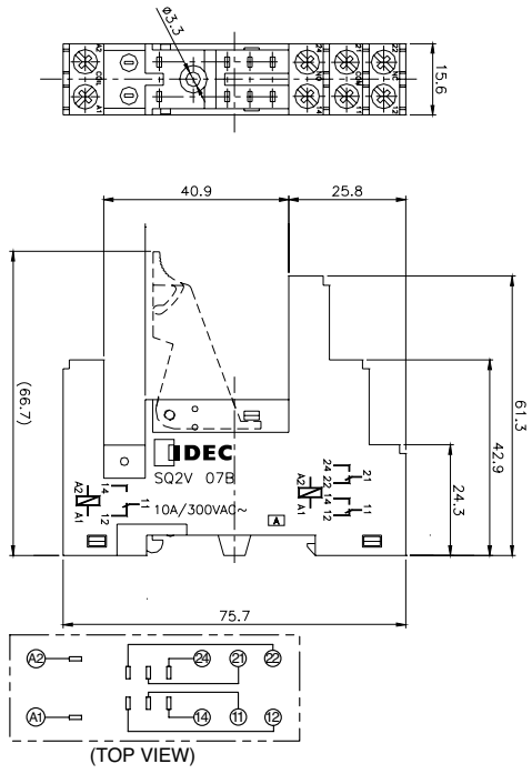
SQ2V-07B
