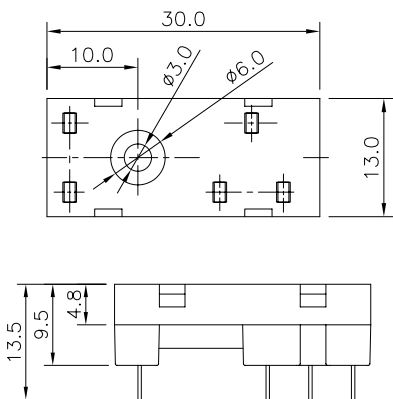
SQ1V-63
