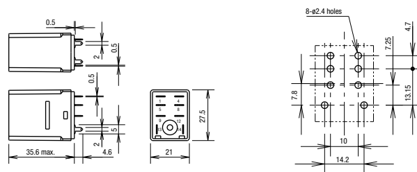
RH4V2-U/RH4V2-UL/RH4V2-UD
