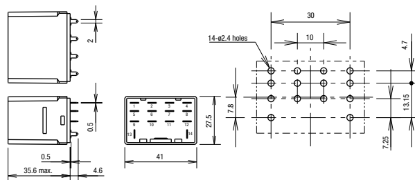
RH4V2-U/RH4V2-UL/RH4V2-UD
